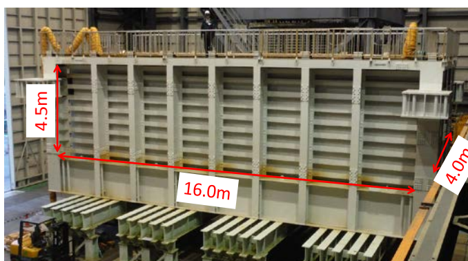
写真-3 直方体剛体土槽
