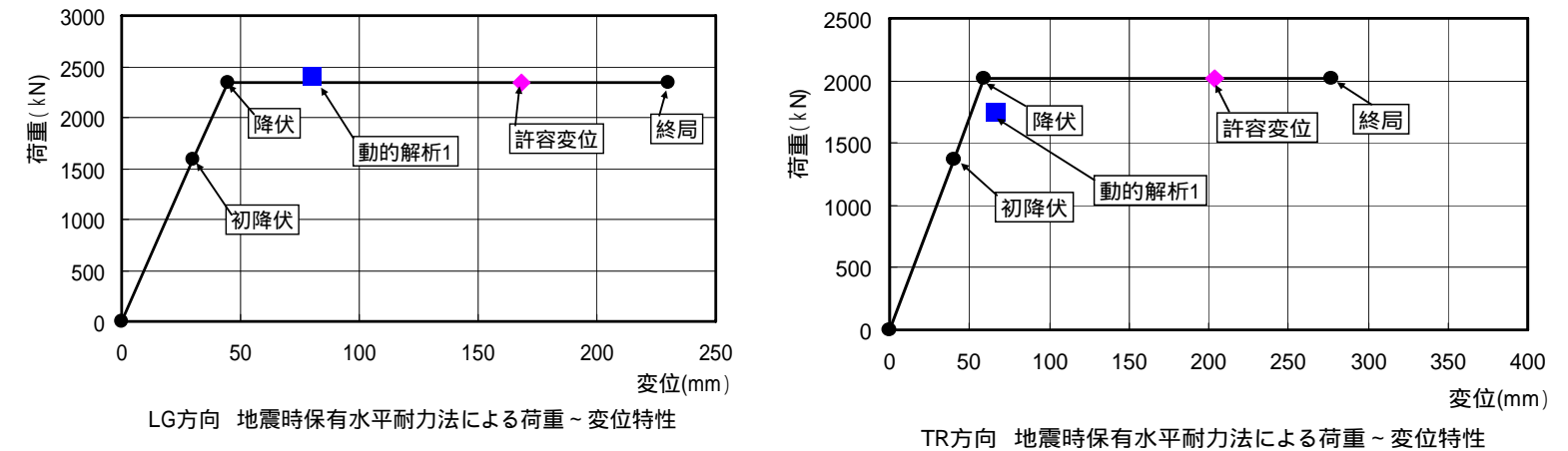
図-2 変形性能
