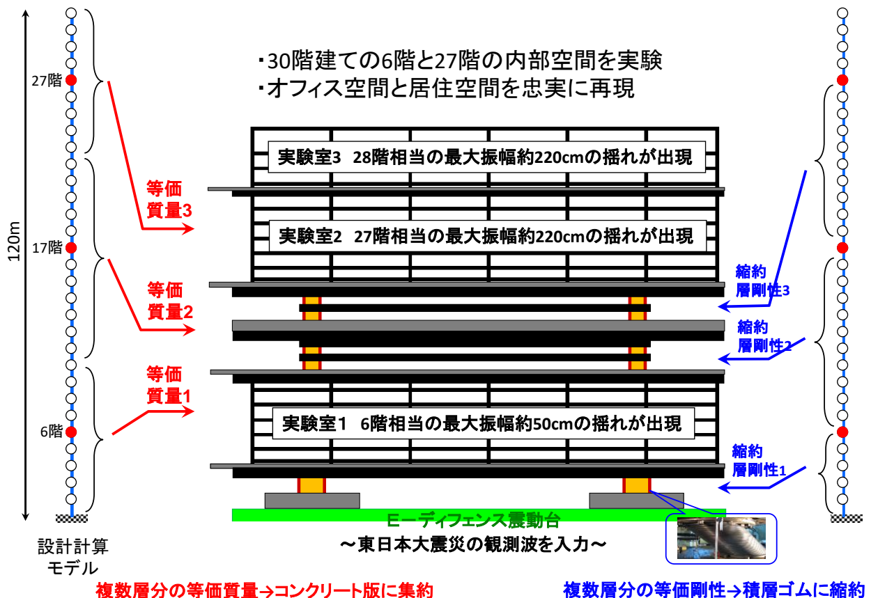
図1 高層建物の設計計算モデルを用いた試験体のモデル化と実験概要
