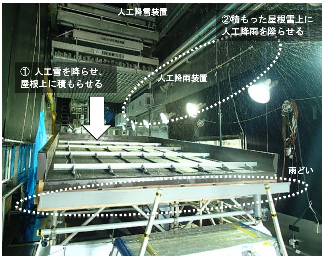
図1 新庄雪氷環境実験所の雪氷防災実験棟内に設置した 仮屋根試験体（幅2.7m、スパン長5m、傾斜2°）と実験の概要
