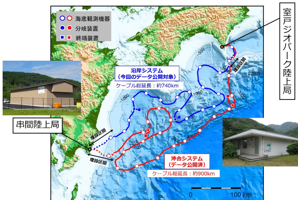
図 N-net 観測点配置図
