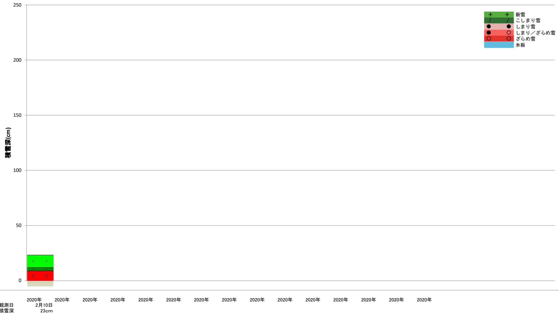
雪氷防災研究センター(長岡)_雪質変化図_2019-2020冬期
