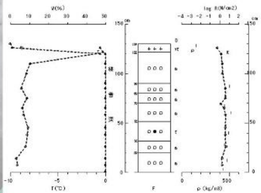
図 No. 積雪断面観測結果 ('2011/03/03 長岡・露場)
