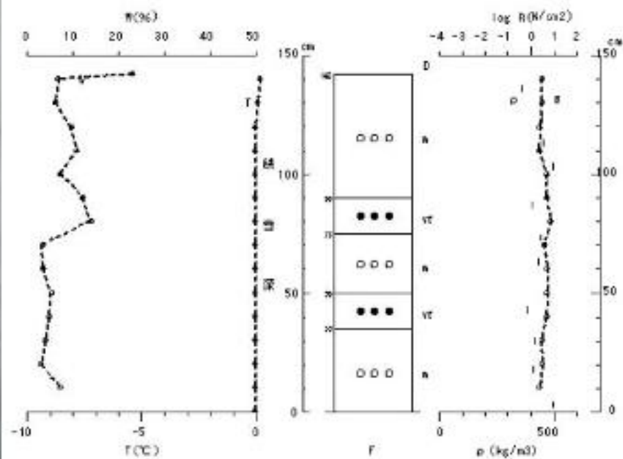
図 No. 積雪断面観測結果 ('2011/02/24 長岡・露場)
