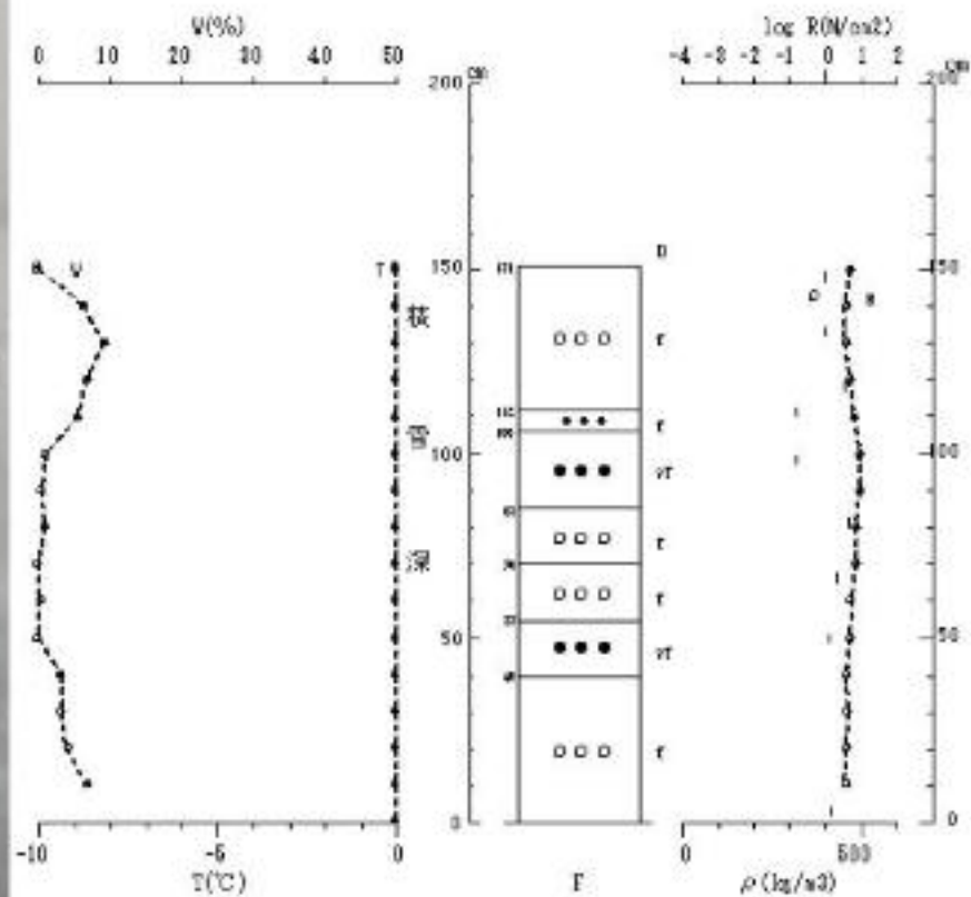
図 No. 積雪断面観測結果 ('2011/02/10 長岡・露場)
