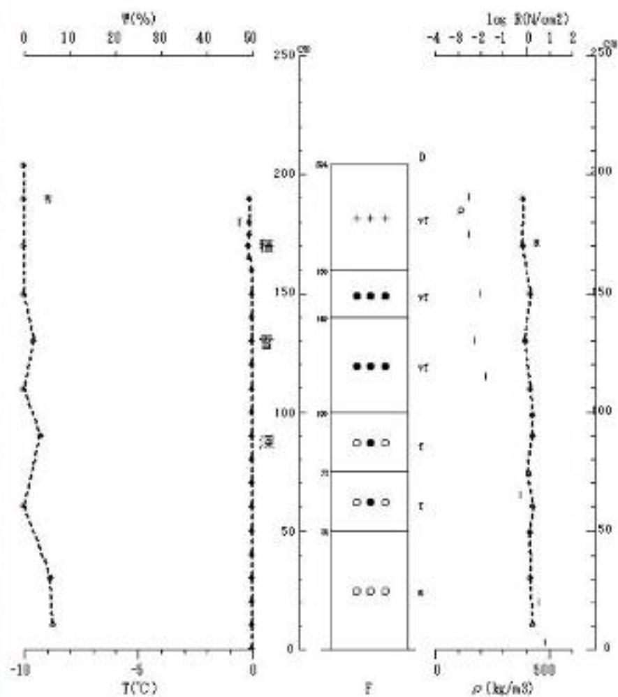
図 No. 積雪断面観測結果 ('2011/01/27 長岡・露場)
