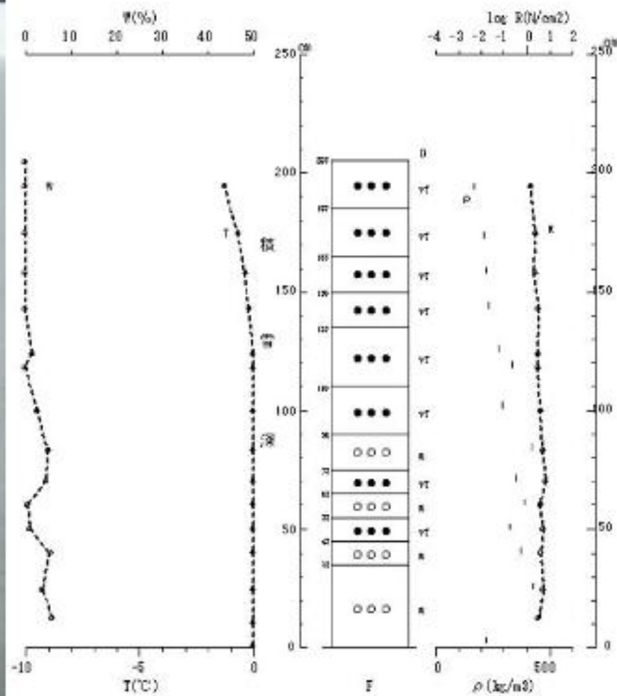
図 No. 積雪断面観測結果 ('2011/02/03 長岡・露場)
