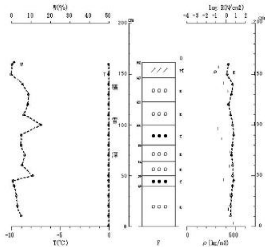
図 No. 積雪断面観測結果 ('2011/02/17 長岡・露場)
