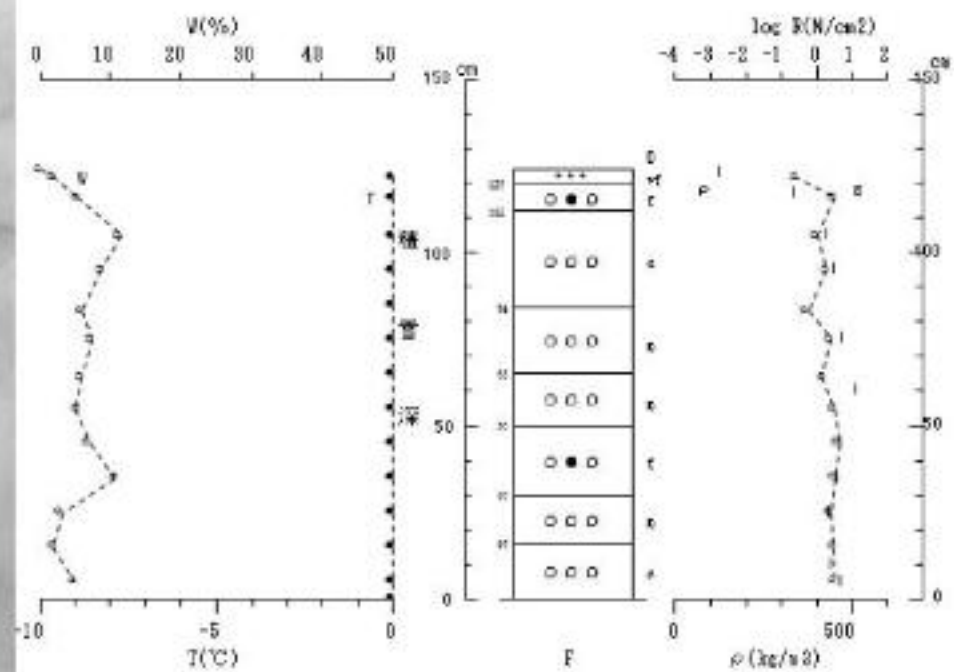
図 No. 積雪断面観測結果 ('2011/03/17 長岡・露場)
