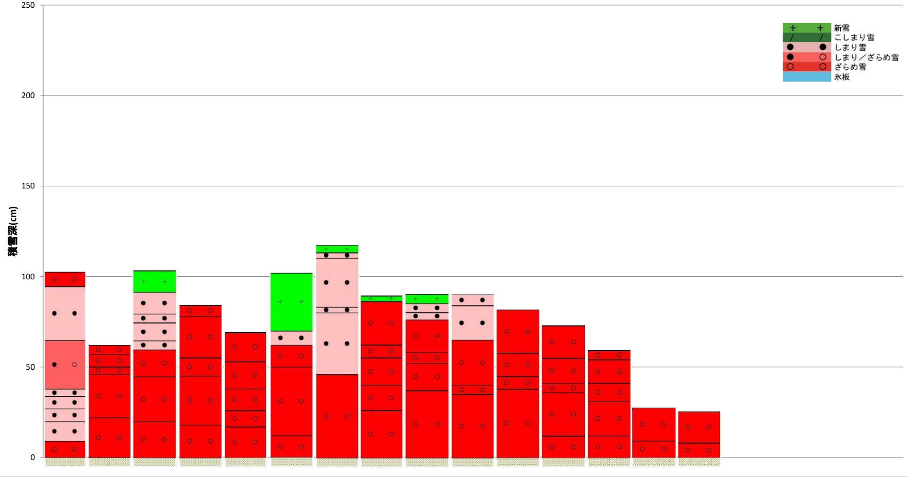
雪氷防災研究センター(長岡)_雪質変化図_2022-2023冬期
