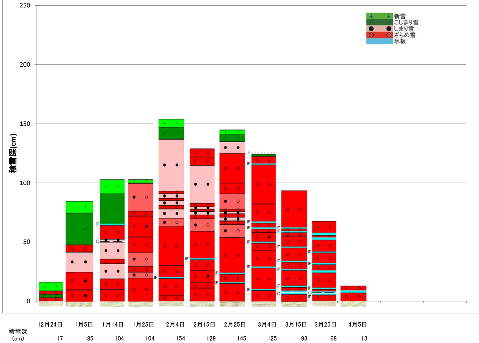
雪氷防災研究センター新庄雪氷環境実験所_雪質変化図_2021-2022冬期
