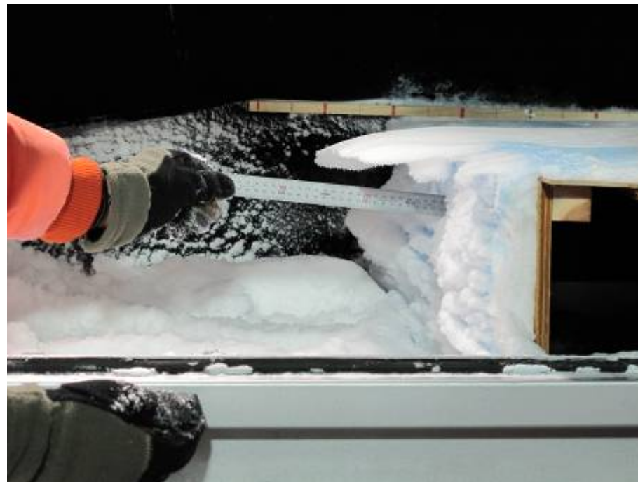
雪庇の形成
