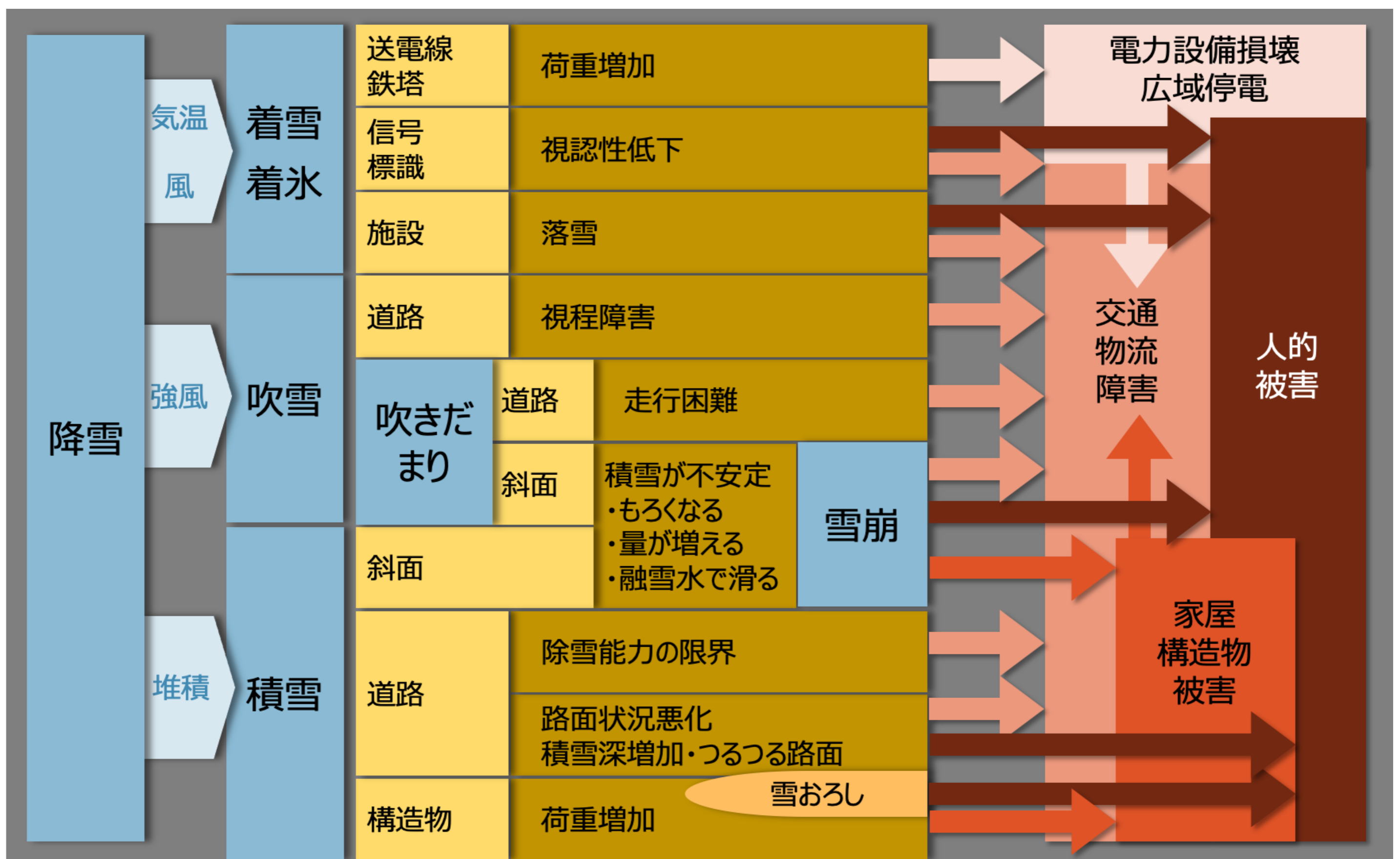
図 雪氷災害イベントツリー
